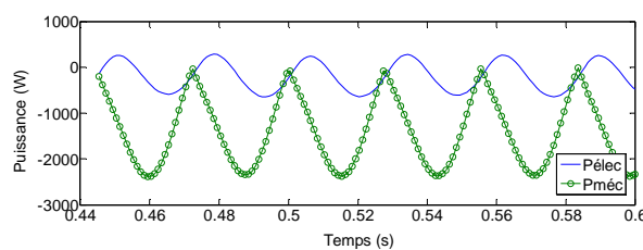
Figure 5 Puissances
