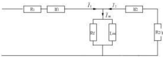
Figure 3 Schéma équivalent
