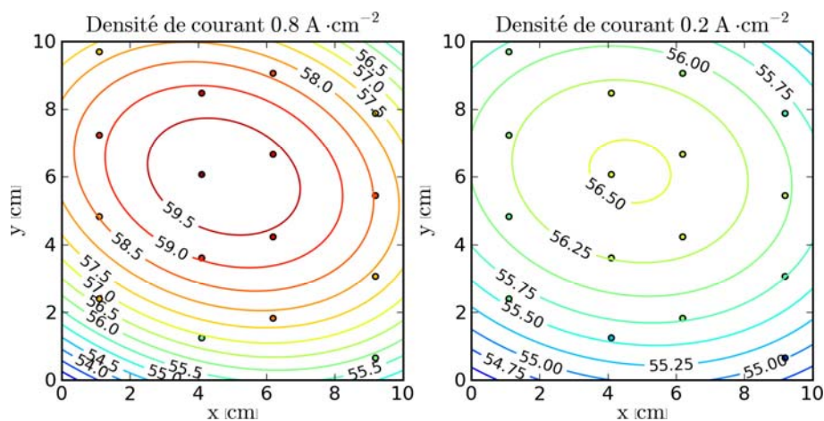
Figure 6 : Cartographie des températures pour 0,8 \text{ A}\cdot\text{cm}^{-2} ( \Delta T = 0,5^\circ\text{C} entre les courbes), et 0,2 \text{ A}\cdot\text{cm}^{-2} de densité de courant ( \Delta T = 0,25^\circ\text{C} entre les courbes).
