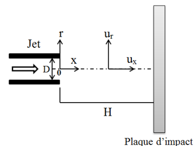
Figure 3 : Position du jet, de la plaque d'impact et direction des composants de la vitesse
