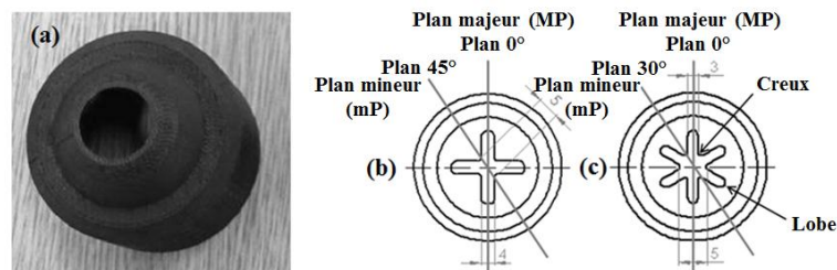
Figure 1 : (a) injection ronde, (b) injection en croix, (c) injection constituée de 6 pétales
