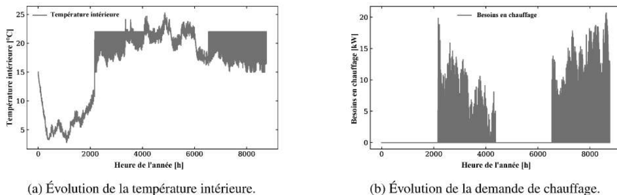
Figure 3 : Résultats de la simulation TRNSYS pour le bâtiment fictif.
