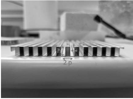
Figure 5 : Dimensions caractéristiques des ailettes
