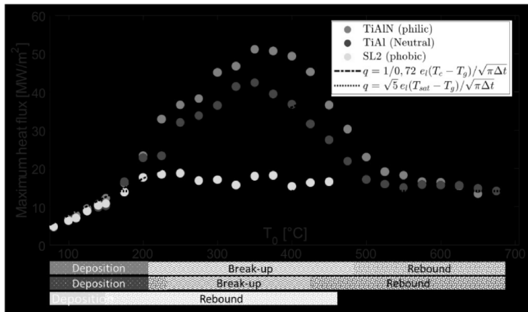
Figure 4. Densité de flux maximale relevée lors de l'impact en fonction de la température initiale de la paroi et de la mouillabilité, model de [5] et [8]
