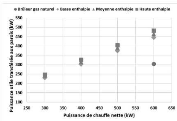
Figure 11 : Puissance utile transférée à l'enceinte en fonction de la puissance nette.
