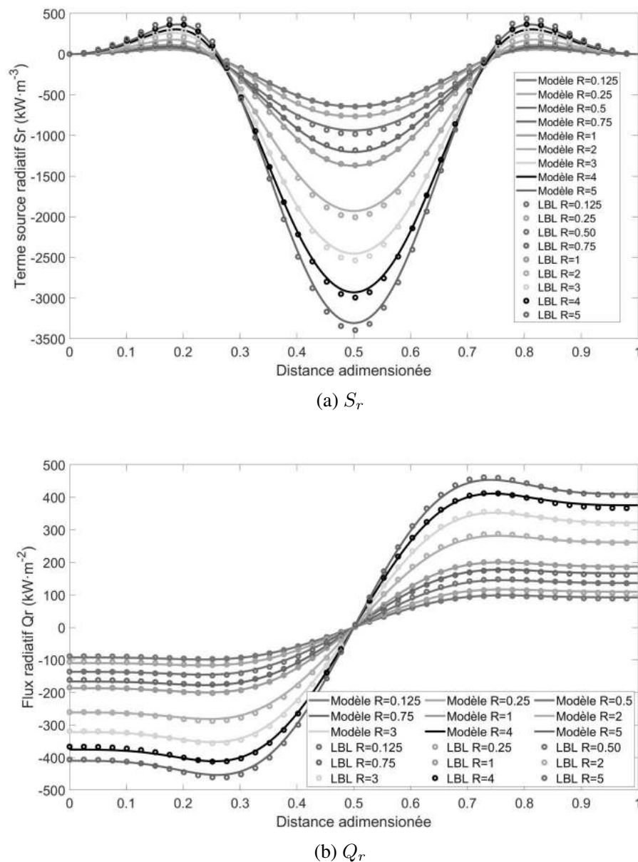
Figure 1 : Comparaison des profils de S_r et Q_r entre le nouveau modèle et la méthode LBL pour un cas test représentatif et pour différentes valeur de R
