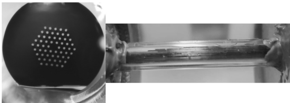
Figure 1 : Échantillon utilisé dans ce travail. Gauche : extrémité d'une fibre et ses 60 microcanaux de diamètre 5.95\mu\text{m} ; droite : monolithe de 60 fibres de 5.9 cm de longueur fixé entre deux échangeurs sur le banc d'essais.
