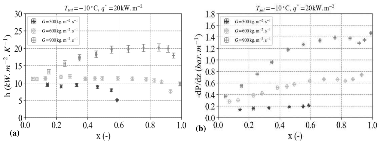
Figure 3 : Evolution du coefficient d'échange thermique et du gradient de pression en fonction du titre vapeur pour différent flux massique: (a) coefficient d'échange thermique et (b) gradient de pression
