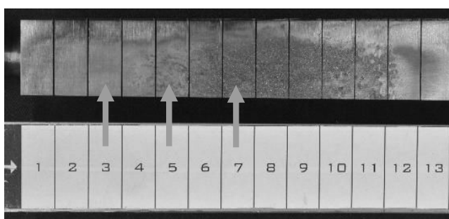
Figure 1 : Position de 14 monoblocs sur le CFP n°270
