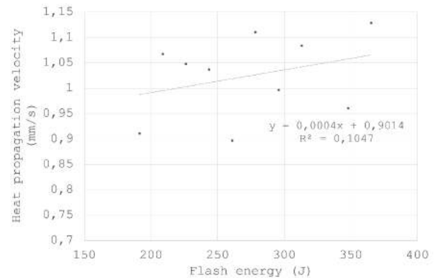
Figure 8 : Vitesse de propagation du front de température en fonction de l'énergie du flash solaire en régime stable, à puissance solaire constante
