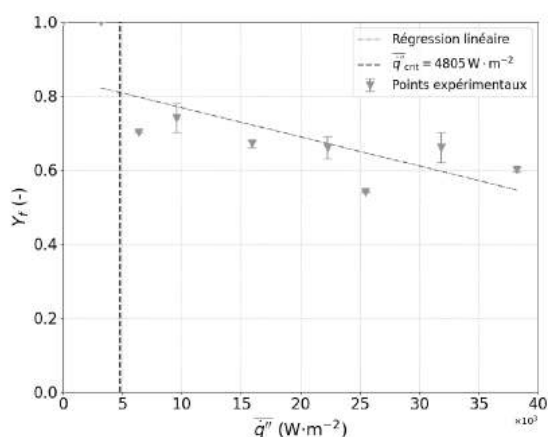
Figure 6 : Fraction massique résiduelle Y_f en fonction \bar{q}'' .
