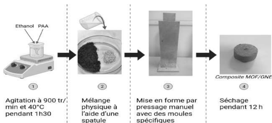
Figure 4 : Préparation du composite MOF/GNE
