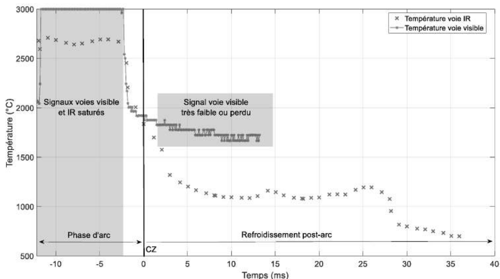
Figure 4 : Thermogrammes IR et visible d'un même essai
