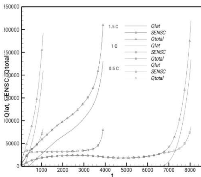
Figure 7: Effet de la vitesse de décharge sur la variation temporelle du stockage de la chaleur
