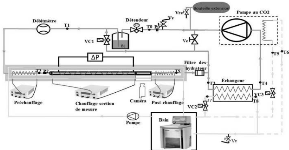
Figure 1 : Vue schématique de l'installation expérimentale
