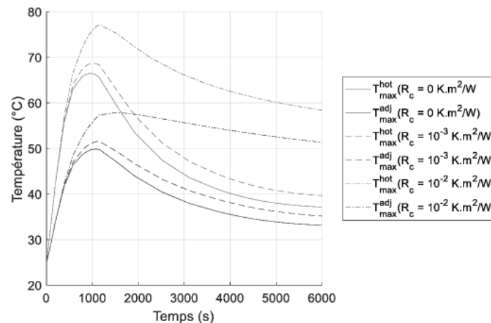
Figure 8 : Comparaison des évolutions temporelles des températures maximales des cellules lors d'une modification du refroidissement du module, en régime dynamique dégradé
