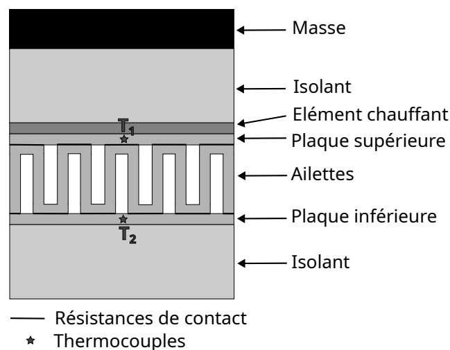
Figure 4 : Schéma de l'expérience
