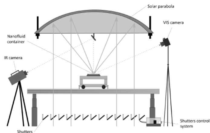
Figure 1 : Schéma du dispositif expérimental
