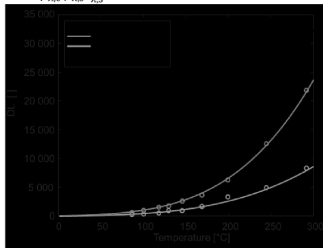
Figure 4 : Comparaison entre les mesures issues de la caméra IR et le modèle
