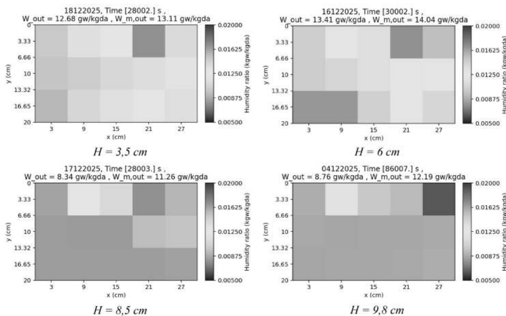
Figure 7 : Répartition locale de l'humidité spécifique en régime permanent selon la hauteur d'imbibition ( Q_v = 10 \text{ L/min} , T_{in} \approx 20^\circ\text{C} , HR_{in} \approx 60 \% , P_{chauffe} = 1 \text{ W} , Protocole : Sec)
