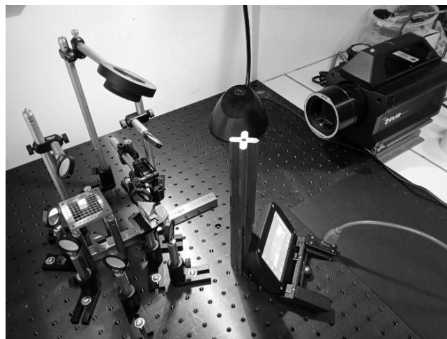
Figure 2 : dispositif expérimental.
