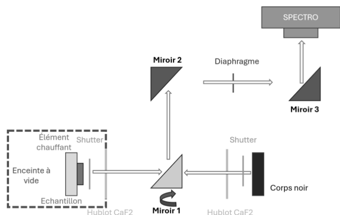
Figure 2 : Schéma de principe du fonctionnement du banc
