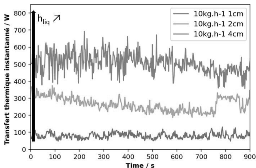
Figure 8 : Comparaison des flux thermiques au fluide secondaire en fonction du temps pour plusieurs hauteurs de liquide. dT_{sat} = 30 K, \dot{m}_{in,fi}=10 kg.h -1 .
