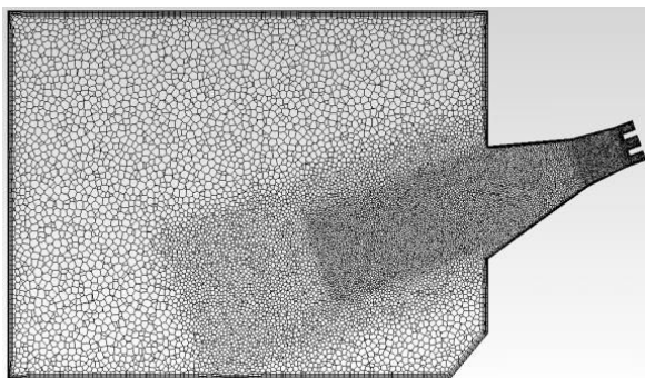
Figure 3 : Maillage cas brûleur
