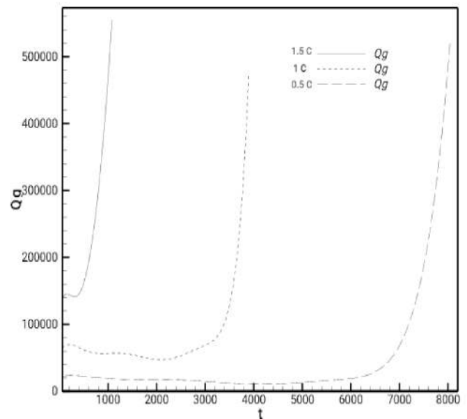
Figure 3: Puissance de chaleur générée en fonction du mode de décharge
