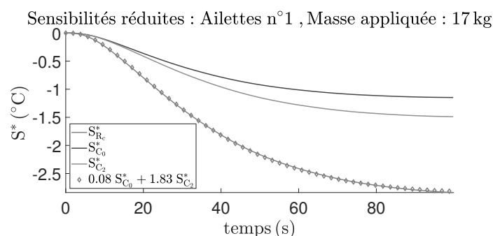
Figure 8 : Sensibilités réduites
