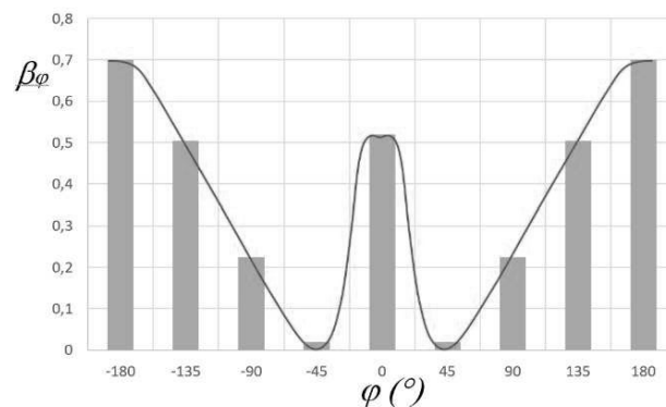
Figure 10 : Rapport \beta_\varphi=(h_w/h_{ref}) en fonction de \varphi
