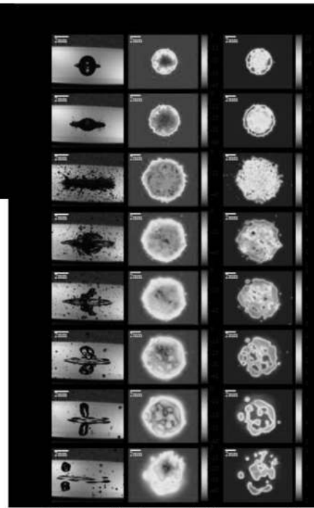
Figure 7 : Impact d'une goutte sur une paroi à T_0=200^\circ\text{C} à We=93
