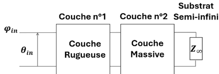
Figure 5 : Représentation quadripolaire du modèle thermique où Z_{\infty} = 1/(b_{\infty}\sqrt{p}) .
