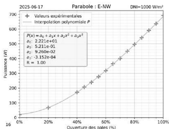
Figure 3 : Puissance du flash thermique en fonction de l'ouverture des obturateurs
