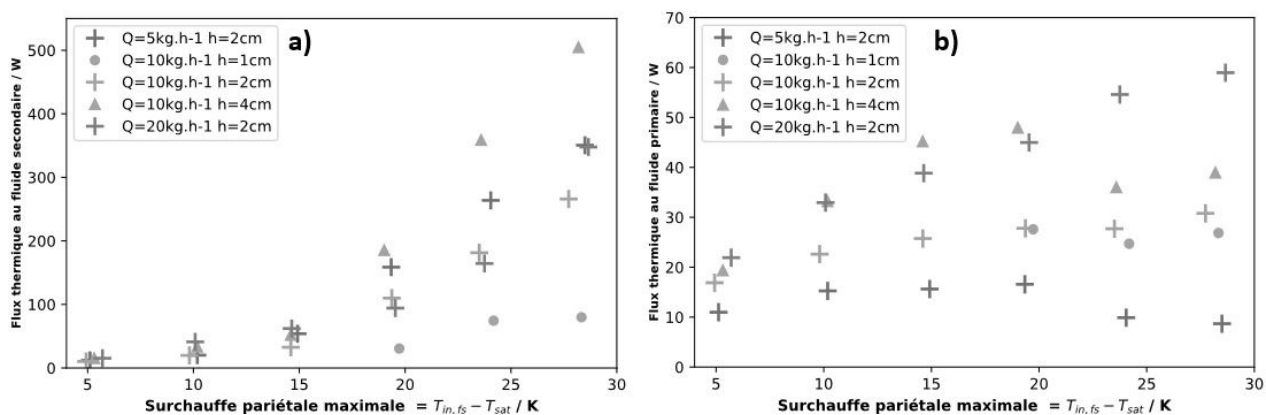
Figure 6 : Flux thermique moyen mesuré au fluide secondaire a), et chaleur sensible gagnée par le fluide de travail b), pour plusieurs configurations et surchauffes pariétales maximales. Par soucis de lisibilité, les incertitudes ne sont pas représentées mais sont équivalentes à celles de la figure 4.
