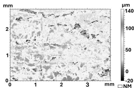
Figure 3 : Topologie de surface du MB n°07
