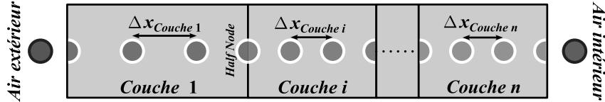
Figure 1: Représentation des nœuds pour un modèle de conduction par différences finies.
