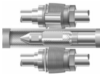
Figure 3-b : Laminage à froid du GEWA-PB
