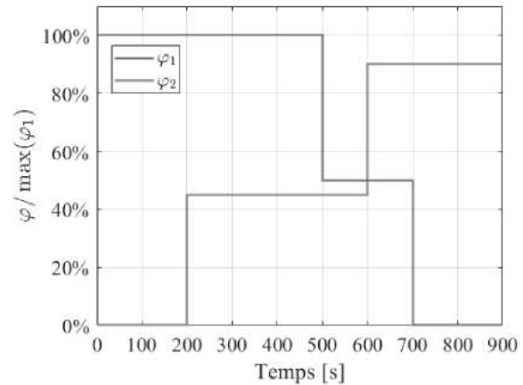
Figure 2 : Evolution temporelle du flux thermique.
