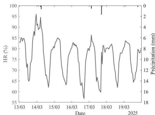
Figure 4 : Evolution de l'humidité relative et des précipitations du 13 au 19 mars.
