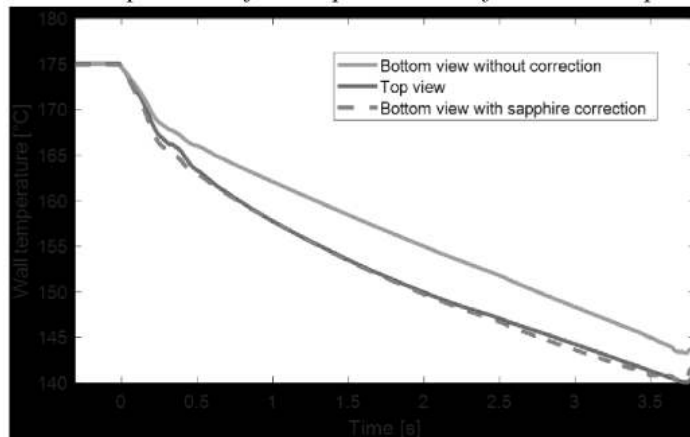
Figure 6 : Evolution de la température du dépôt
