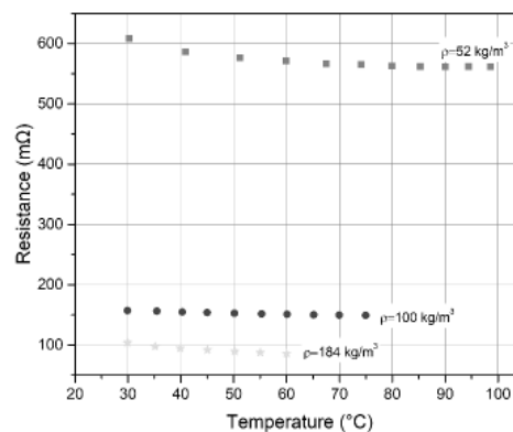
Figure 8 : Variation de la résistance en fonction de la température pour les trois matrices GNE. \rho = 52, 100 et 184 \text{ kg/m}^3 ; I = 7.5 \text{ A} .
