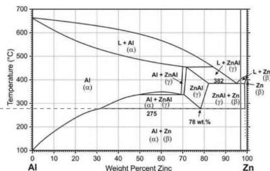
Figure 7: Diagramme de phases de l'alliage Zn-Al
