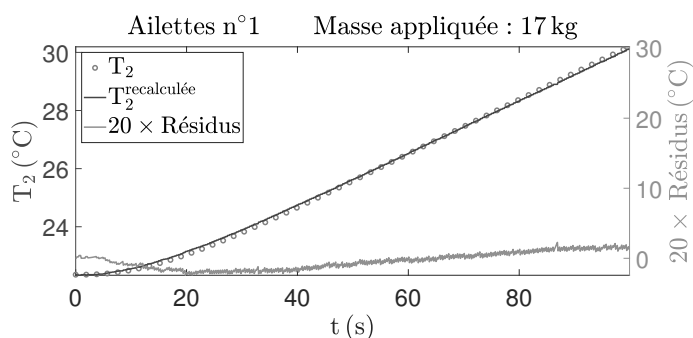
Figure 9 : T_2 recalculée
