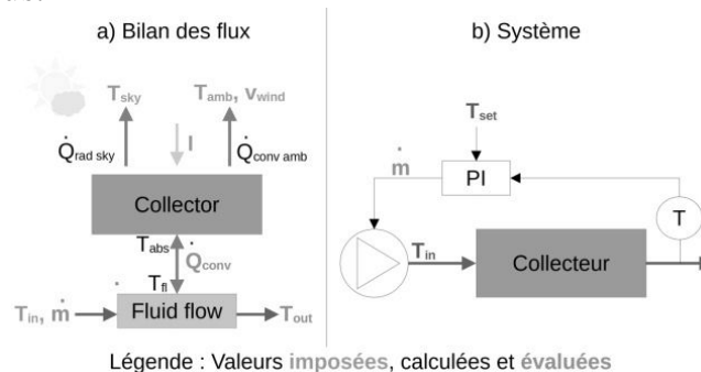
Figure 5 : Schéma de l'étude système du collecteur cylindro-parabolique et son pilotage
