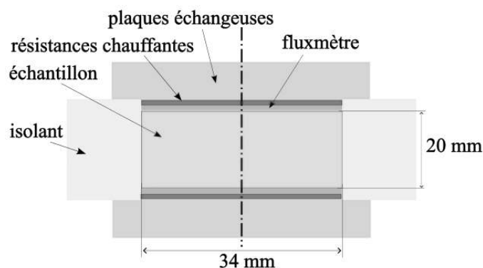
Figure 2 : Dispositif expérimental
