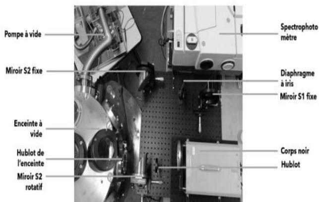
Figure 1 : Photo du banc expérimental
