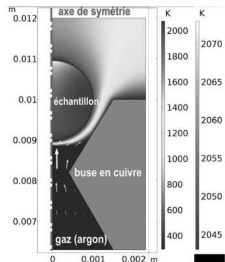
Figure 4 : Champs de température et vecteurs vitesse dans l'argon et l'échantillon issus du modèle, pendant un tir laser ( t = 3 s).
