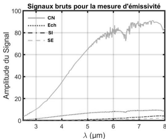
Figure 8 : Signaux bruts de l'échantillon de 1 (référence)
