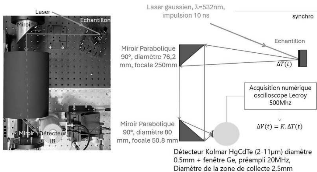
Figure 4. Gauche : Banc expérimental. Droite : Schéma de fonctionnement
