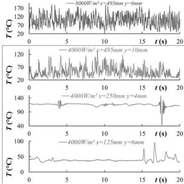
Figure 3 : Instabilités thermiques de couche limite.
