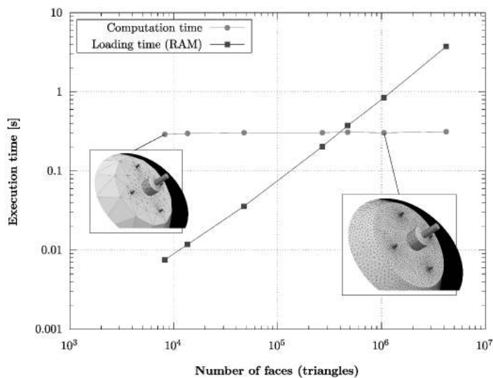
Figure 3 : À gauche : insensibilité du temps de calcul du flux radiatif moyen (avec \pm 1\% d'incertitude) reçu par la sole d'une chambre de combustion en fonction du raffinement géométrique. À droite : visualisation des chemins optiques des photons à l'intérieur du four. Certains photons sont réfléchis ou absorbés par les parois, d'autres sont absorbés par les gaz d'enceinte. Les calculs ont été réalisés avec RadForceE sur un processeur Intel Core i5-1145G7 (1 cœur, 2 threads actifs, 4 GHz).
