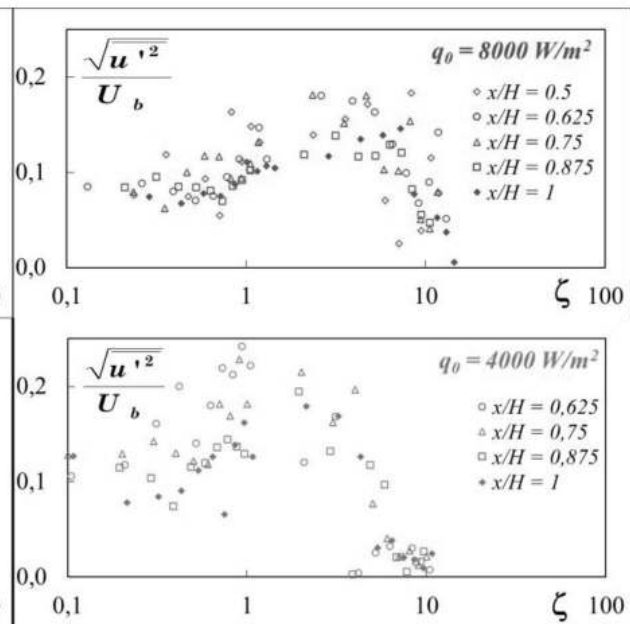
Figure 8 : Intensité turbulente dynamique.
