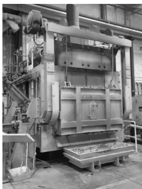
Figure 1 : Photo du four réverbère équipé d'un brûleur gaz naturel (configuration actuelle).
