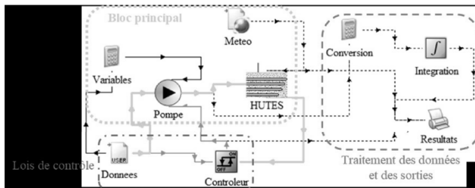
Figure 2 : Modélisation sous TRNSYS d'un HUTES (scénario 3)
