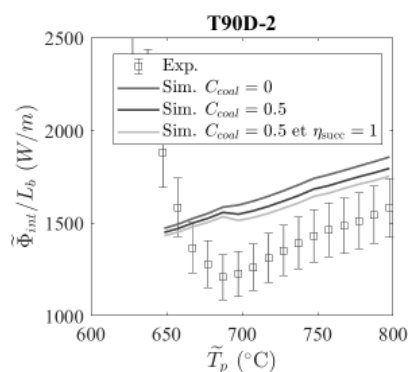
Figure 6 : Comparaison du flux thermique expérimental (T90D-2) et numérique pour le cas de coalescence idéaliste ( \eta_{\text{succ}} = 1 , C_{\text{coal}} = 0.5 ).
