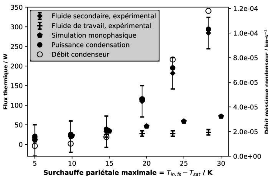
Figure 4 : Comparaison des flux thermiques expérimentaux échangés par le fluide secondaire et le fluide de travail, et simulé sans changement de phase. h_{\text{liq}}=2 cm et \dot{m}_{\text{in,ft}}=10 kg.h -1 .
