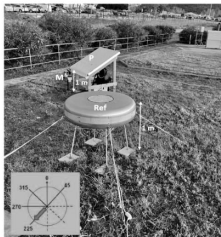
Figure 3: Photographie du condenseur incliné à 30^\circ (P, direction SW) et du condenseur horizontal. Légende de la rose des vents: direction du vent la nuit (flèche noire) et l'angle des orientations testées
