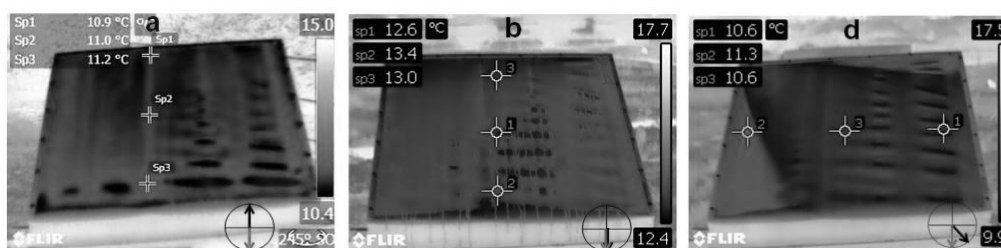
Figure 6: Température de surface pour différentes orientations \varphi du vent. Orientation: flèche blanche orientation du condenseur, flèche noire direction du vent. (a) \varphi = 180^{\circ} , 3/10/2023, 03:20, U_1 = 2.2 m \cdot s^{-1} . (b) \varphi = 0^{\circ} , 10/09/2023, 04:10, U_1 = 2 m \cdot s^{-1} . (c) \varphi = 45^{\circ} , 27/09/2023, 04:10, U_1 = 2.2 m \cdot s^{-1} .
