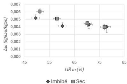
Figure 6 : Variation de l'humidité spécifique sortie entrée selon HR_{in} et selon le protocole utilisé ( Q_v = 10 \text{ L/min} , H = 5,5 \text{ cm} , T_{in} \approx 20^\circ\text{C} , P_{chauffe} = 1 \text{ W} )
