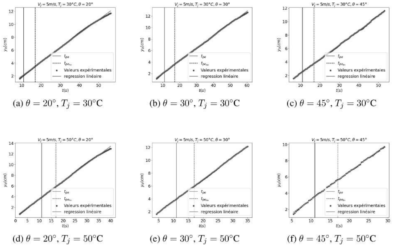
Figure 5 : Régression linéaire sur les courbes y_0(t) pour V_j = 5 \text{ m/s} , et T_j \in \{30^\circ\text{C}, 50^\circ\text{C}\} , avec inclinaisons \theta \in \{20^\circ, 30^\circ, 45^\circ\} .
