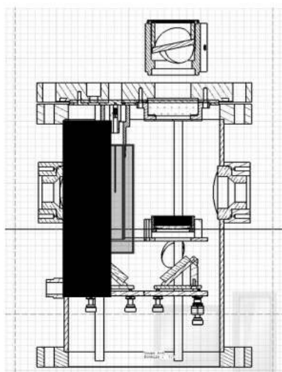
Figure 1 : Plan de l'installation G124-18 Laser
