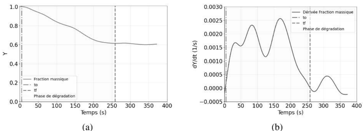
Figure 4 : Évolution de la fraction massique (a) et de sa dérivée (b) pour une densité de flux externe de 38196 W·m -2 .
