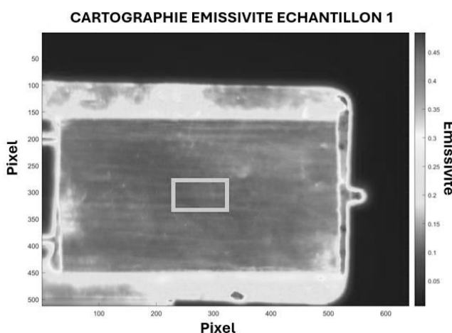
Figure 7 : Cartographie de l'émissivité de l'échantillon 1 (référence)
