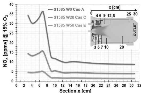
Figure 3 : Evolution de la concentration en \text{NO}_x dans la chambre de combustion pour des syngaz à haute teneur en vapeur d'eau
