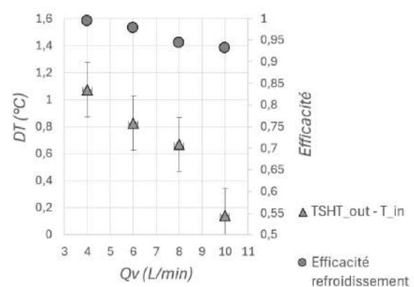
Figure 9 : Influence du débit d'air sec en entrée sur la différence de température sortie/entrée de la veine et le potentiel de refroidissement de l'air humide dans le canal ( T_{in} \approx 19^\circ\text{C} , H = 3,5 cm, HR_{in} \approx 70\% , P_{chauffe} = 1 W, Protocole : Sec)
