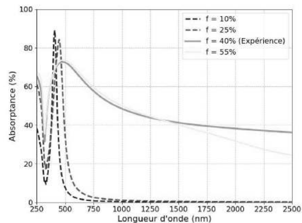
Figure 6 : Influence de la fraction volumique métallique f sur l'absorptance spectrale avec ( d = 53 nm, r = 5 nm, L = 0.44 ).
