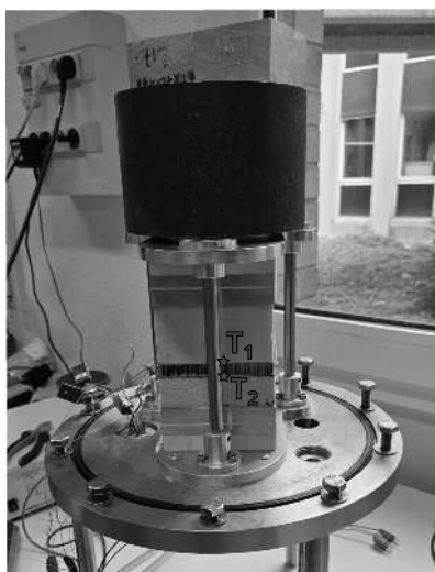
Figure 3 : Installation expérimentale
