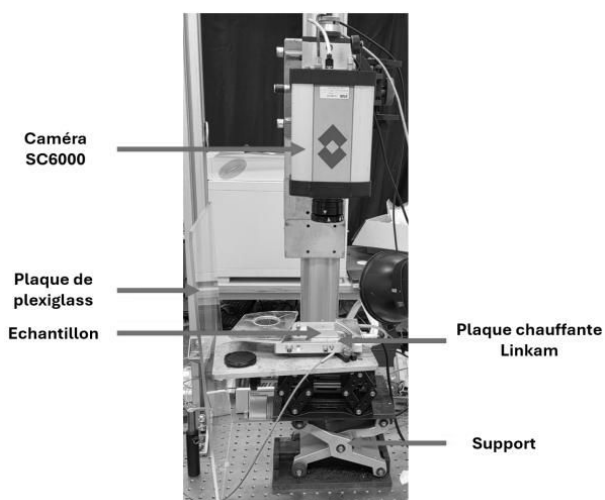
Figure 6 : Photo du banc expérimental avec caméra IR
