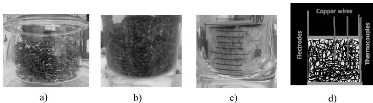
Figure 1 : Montage de l'unité de stockage
