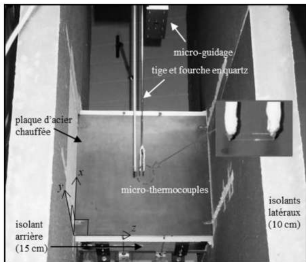
Figure 1 : Dispositif métrologique.
