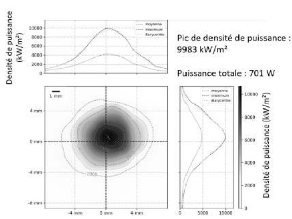
Figure 2 : Caractérisation de la parabole au point focal
