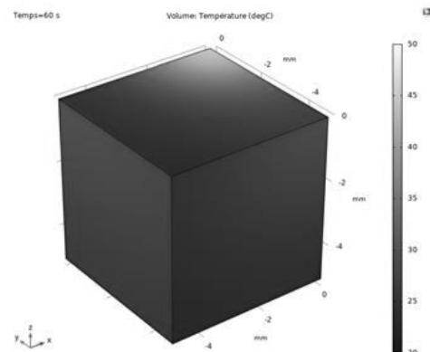
Figure 11 : champ de température à t = 60 \text{ s} .
