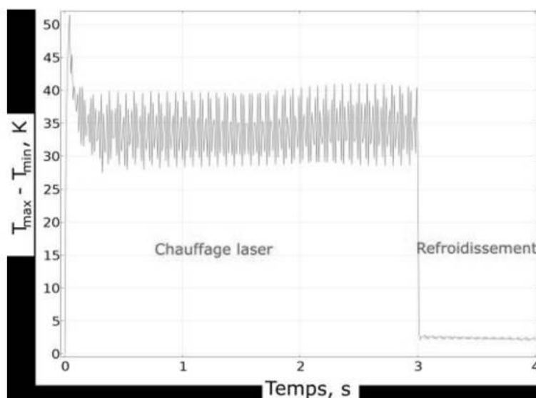
Figure 3 : Différence entre les températures maximales et minimales dans la goutte. Le laser est coupé à 3 secondes.
