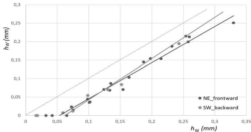
Figure 9 Correlation entre ( h_w ) and ( h_w' ) pour un vent de face(en rouge) et un vent arrière (en bleu). La ligne pointillé est la droite de pente 1.
