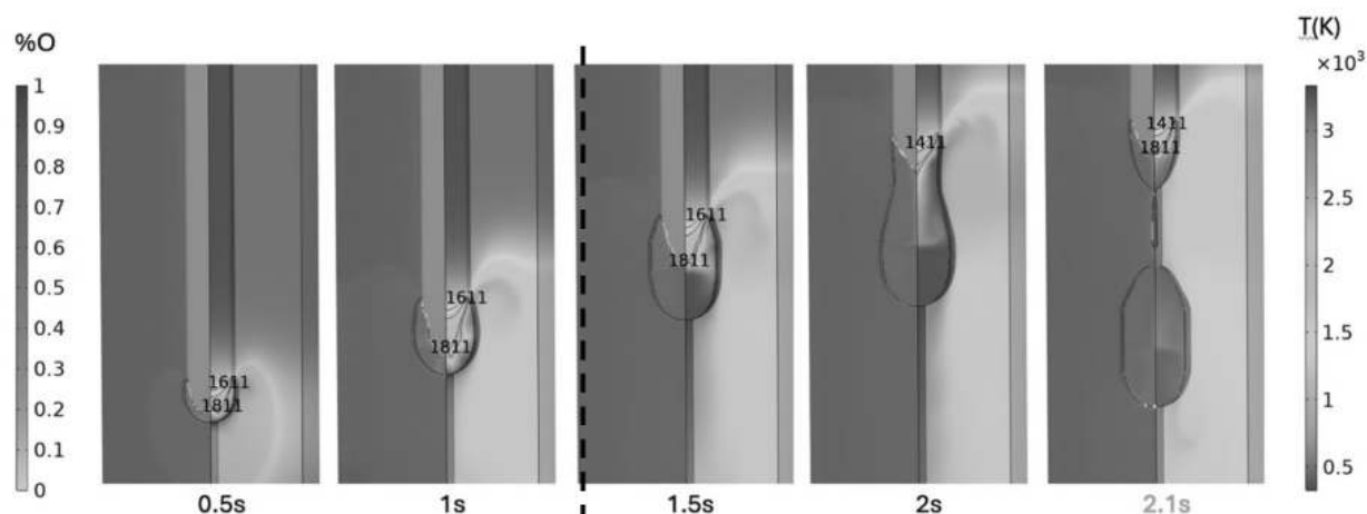
Figure 3 : Comportement géométrique durant la combustion (Laser : 1000W -1s-diamètre 2mm).
