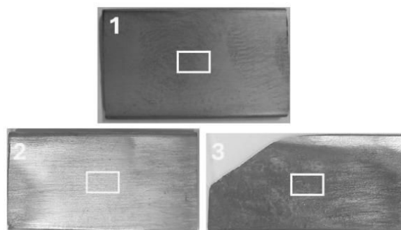
Figure 5 : Échantillons provenant de la machine : 1) référence – 2) zone érodée – 3) zone de dépôts
