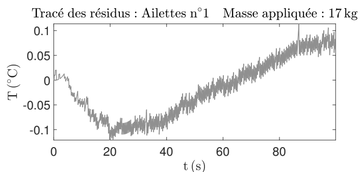
Figure 10 : Résidus
