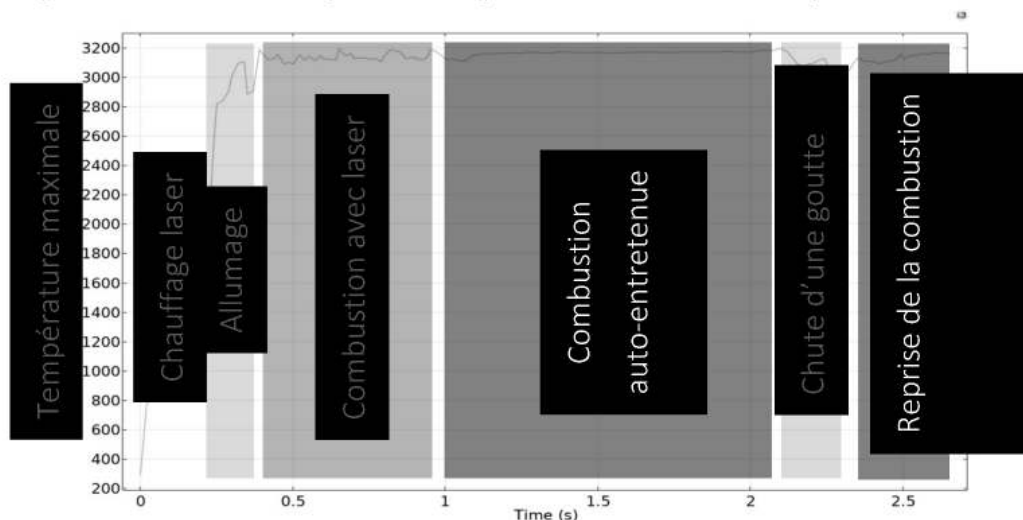
Figure 4: Comportement thermique du barreau (Laser : 1000W -1s-diamètre 2mm)
