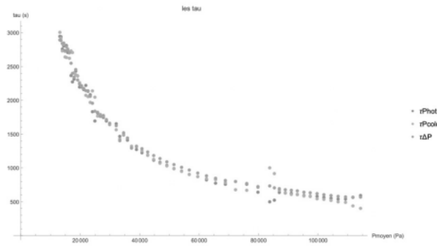
Figure 3 : Temps caractéristique des écoulements pour la mesure de perméabilité. 3 mesures utilisant respectivement le fit de la pression coté chaud, coté froid et de la différence de pression sont présentées ici et comparées. Les résultats sont identiques
