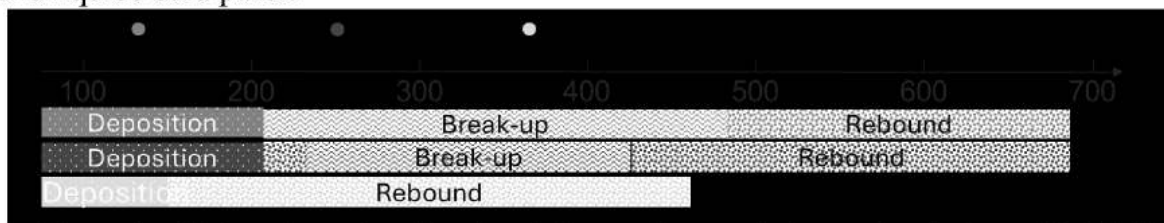
Figure 3 : Régime observé en fonction de la température de la paroi et de la mouillabilité
