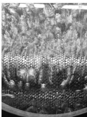
Figure 4-b : GEWA-PB pour un \Delta T de 2K
