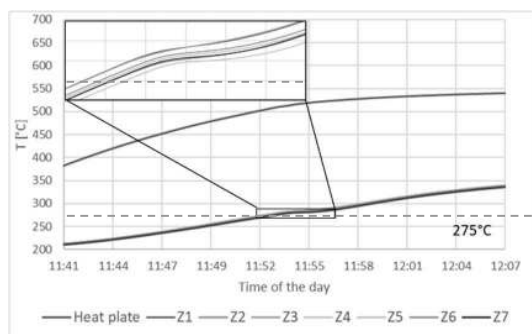
Figure 6: Température mesurées dans le bloc de Zamak
