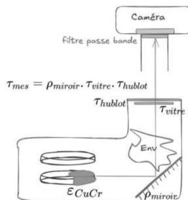
Figure 2 : Système optique des contacts jusqu'aux caméras
