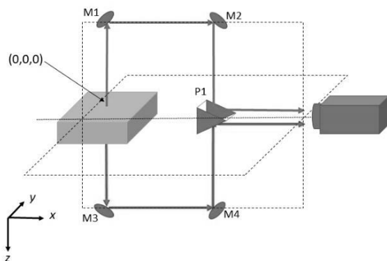
Figure 3 : Schéma du dispositif expérimental [13].
