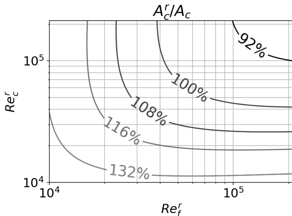
Figure 3 : Gain de compacité avec les TPMS
