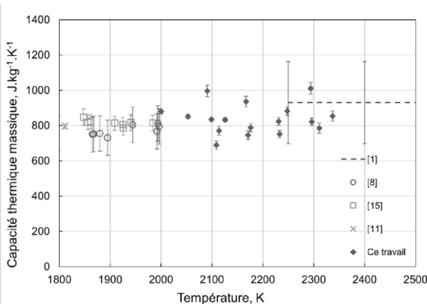
Figure 5 : Capacité thermique massique du fer liquide comparée à la littérature.
