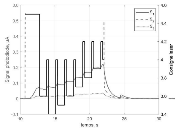
Figure 7 : Données brutes pour un test sur un échantillon de fer.
