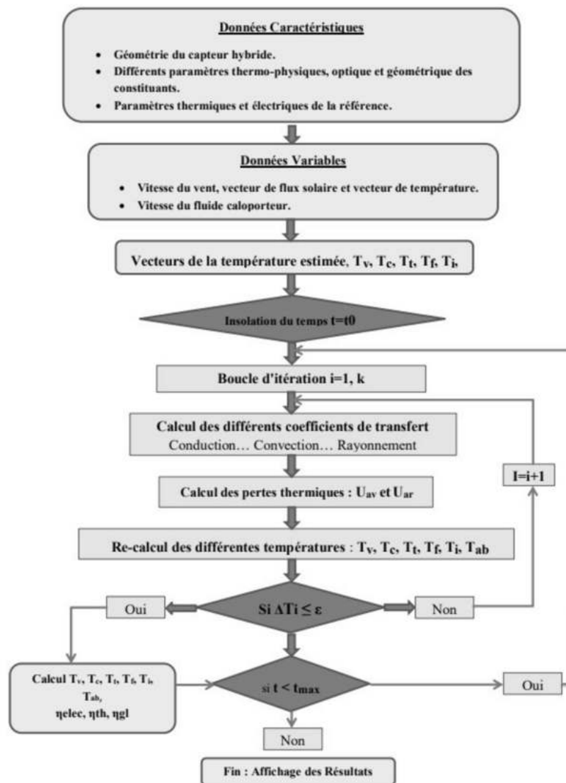
Figure 2 : Diagramme de résolution numérique du système PV/T
