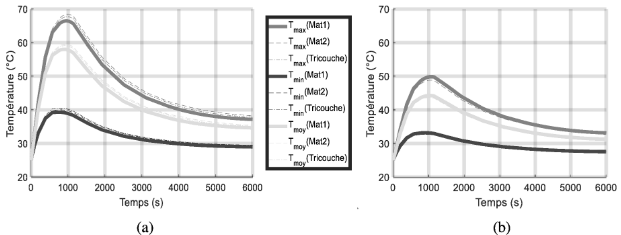
Figure 6 : Comparaison des évolutions temporelles des températures des cellules en régime dégradé pour les trois matériaux testés : (a) Cellule sursollicitée (b) Cellule adjacente
