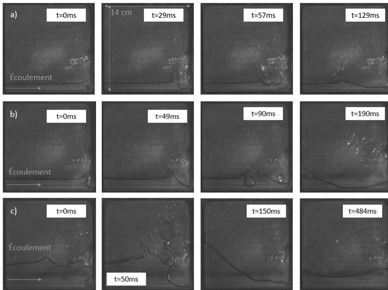
Figure 7 : Évènements typiques d'ébullition observés pour a) h_{liq}=1 cm, b) h_{liq}=2 cm et c) h_{liq}=4 cm. P=10 mbar, dT_{sat}=30 K et \dot{m}_{in,fi}=10 kg.h -1 . Les temps sont donnés à titre indicatifs.
