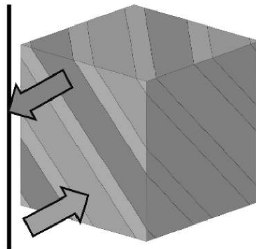
Figure 2 : Maille élémentaire fluides d'échangeur Schwarz-Diamant
