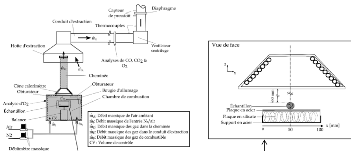
Figure 2 : Dispositif expérimental.
