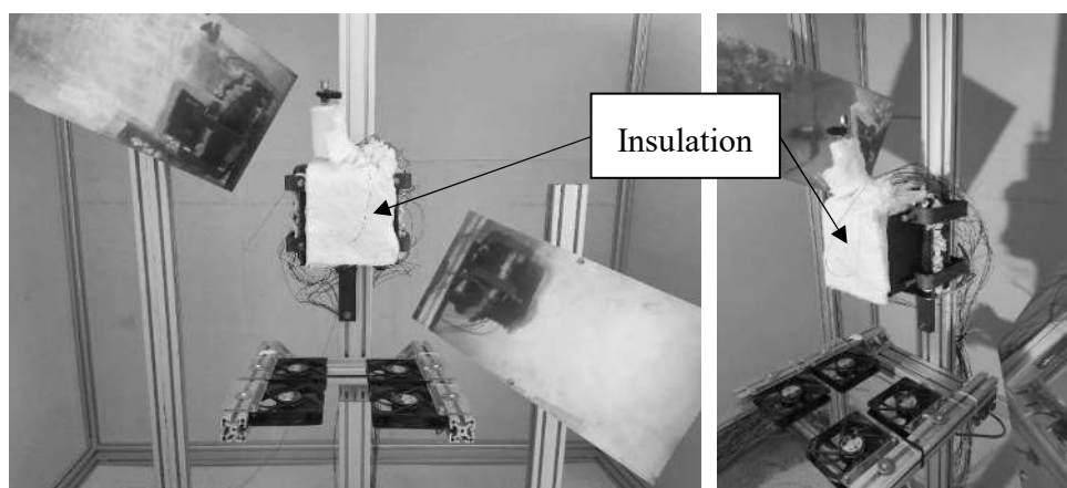
Figure 3: Photos du dispositif expérimental Zabox
