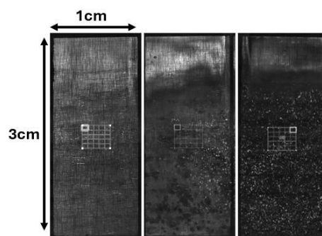
Figure 2 : Aspect de surface des monoblocs n°03, 05 et 07
