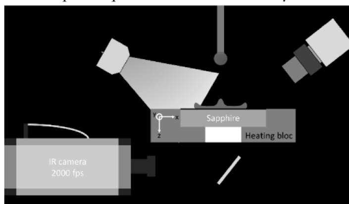
Figure 1: Dispositif expérimental utilisé
