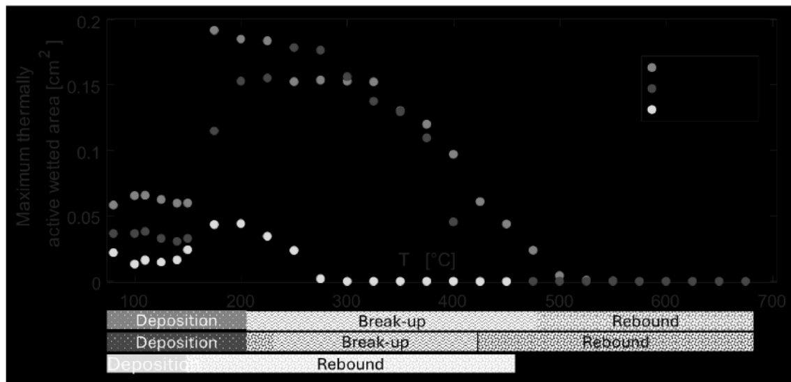
Figure 5 : Surface maximale thermiquement active en fonction de la température initiale et de la mouillabilité
