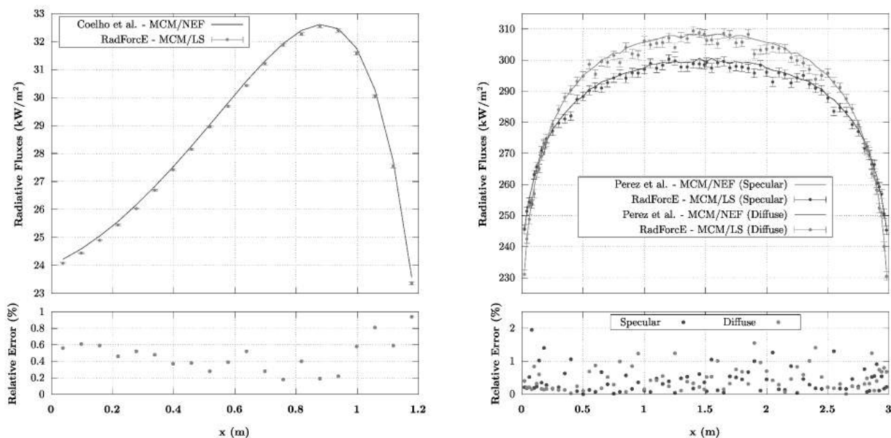
Figure 2 : Comparaison des flux de chaleur calculés avec RadForceE (données spectroscopiques HI-TEMP2010 [11]). À gauche : cas hétérogène avec parois noires ( N = 1\,000\,000 réalisations MC/point, \mathbb{D}_\nu \in [300, 10\,000] \text{ cm}^{-1} ), comparé à la méthode de Coelho et al. [9]. À droite : cas homogène avec parois réfléchissantes ( N = 40\,000 réalisations MC/point, \mathbb{D}_\nu \in [0.1, 12\,500] \text{ cm}^{-1} ), comparé à la méthode de Perez et al. [10]. Les barres d'erreur représentent un intervalle de confiance de \pm 1\sigma . Sous chaque graphique, l'erreur relative absolue entre les deux modèles est représentée pour chaque point de calcul.
