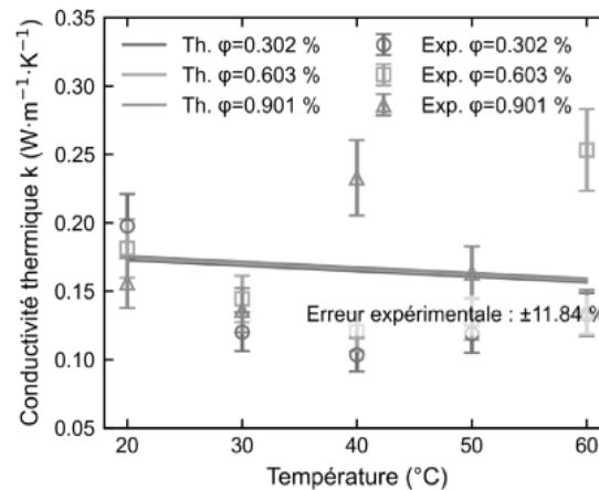
Figure 3 : Conductivité thermique du nanofluide Graphite/éthanol.
