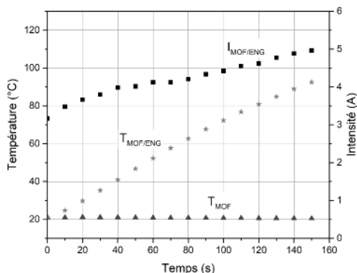
Figure 9 : Variations des températures et du courant pour le MOF et le composite en fonction du temps sous tension continue de 4.6\text{ V} .
