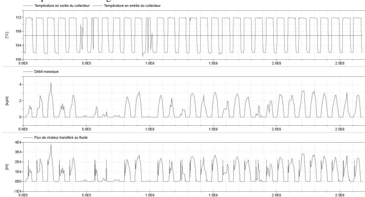
Figure 6 : Résultat du cas de base pour l'analyse système des collecteurs cylindro-paraboliques
