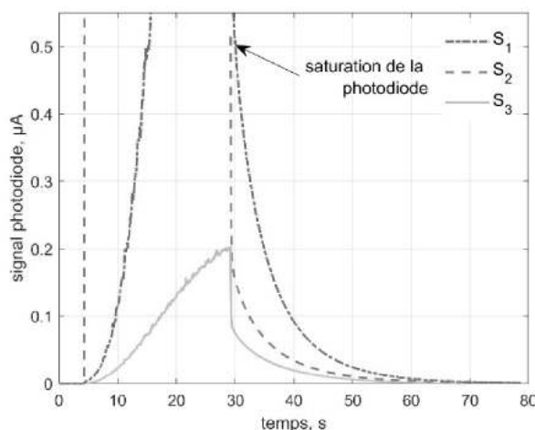
Figure 4 : Signaux bruts S_1 , S_2 et S_3 en fonction du temps durant l'étalonnage.
