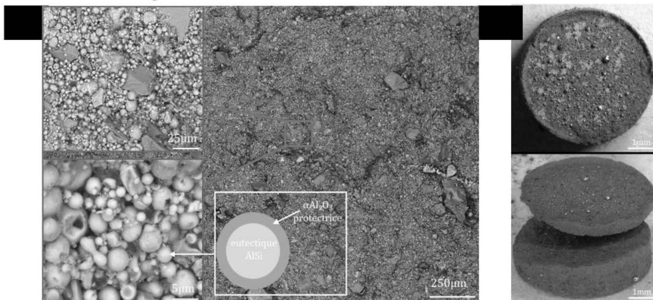
Figure 3 : Images du mélange M1-Al-Si (50 : 50 % massique) après traitement thermique à 600 °C sous air a) en coupe transverse observée au MEB et b) en microscopie optique vu du dessus et de profil.
