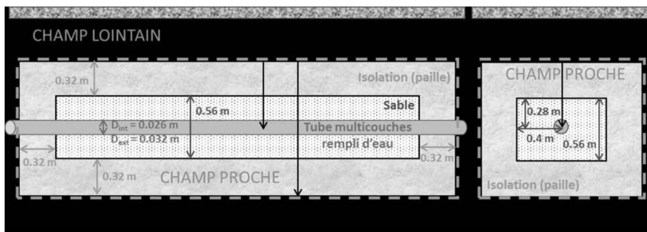
Figure 1 : Schéma simplifié de la vue de côté (plan X-Z) (a) et de la coupe verticale (plan Y-Z) (b)
