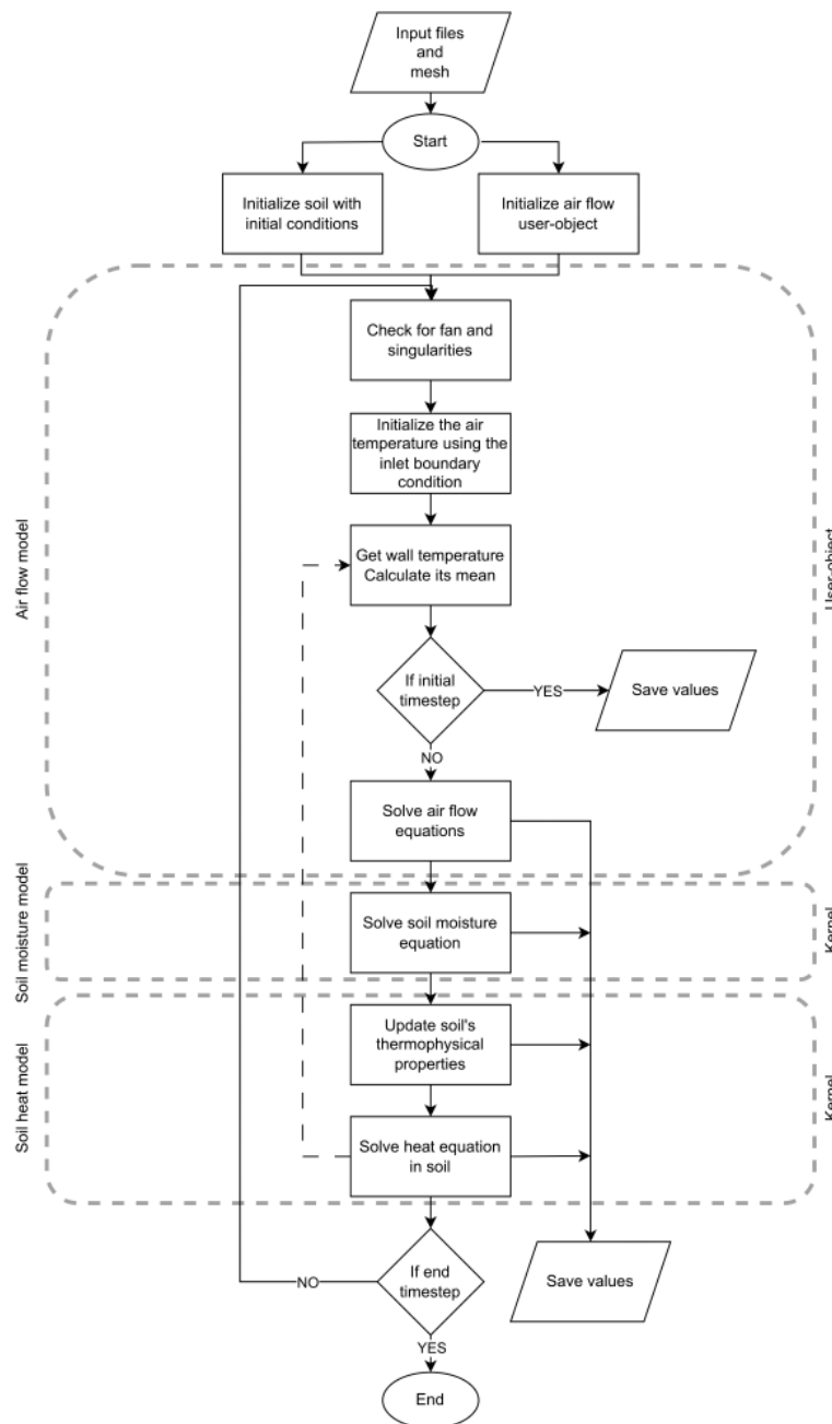
Figure 1 : Algorithme de simulation des échangeurs air-sol (EAHE).
