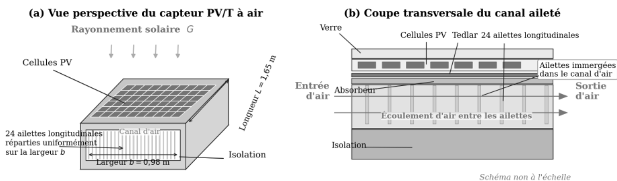
Figure 1 : (a) Vue du capteur PV/T à air avec cellules, canal d'air et 24 ailettes longitudinales. (b) Coupe transversale montrant les couches et l'écoulement d'air entre les ailettes immergées. Schéma non à l'échelle.
