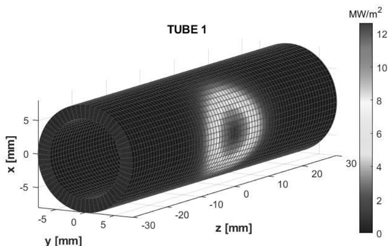
Figure 1 – Cartographie du flux incident « TUBE 1 »
