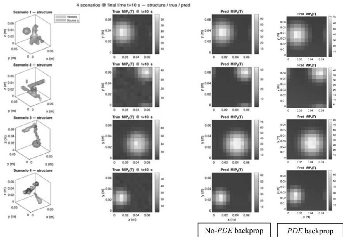
Figure 2 : Comparaison entre la température (vraie = mesurée) utilisée pour l'entraînement du réseau et celle calculée (prédite) par le réseau optimal pour les scénarios 1 à 4 au temps final t = 10s . La position des vaisseaux et de la source dans le domaine est visible sur les figures 3D à gauche pour chaque scénario. Les résultats sont présentés en utilisant soit le mode guidé, soit le mode de rétropropagation PDE complète.
