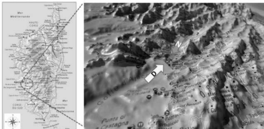
Figure 2: Carte de la Corse et localisation du site expérimental de l'aéroport d'Ajaccio. La flèche jaune indique l'orientation du vent en période diurne (D, orientation SW), les flèches bleues le vent en période nocturne (N, orientation NE).
