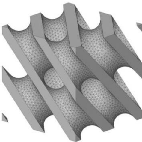
Figure 1 : Maille élémentaire solide d'échangeur TPMS Schwarz-Diamant
