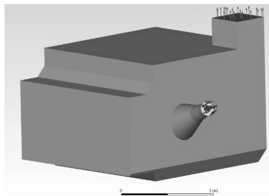
Figure 2 : Simplification géométrie four et volume fluide pour la simulation gaz naturel
