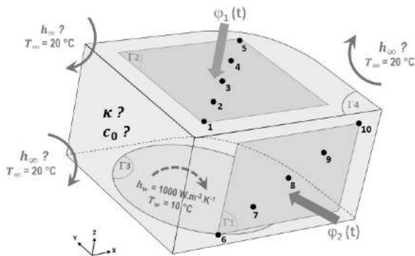
Figure 1 : Géométrie et conditions thermiques retenues pour l'étude.
