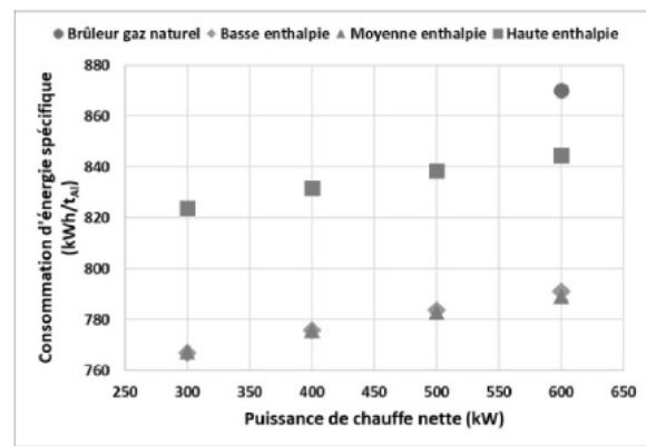
Figure 10 : Consommation d'énergie spécifique estimée pour les différents cas plasma comparée au gaz naturel.
