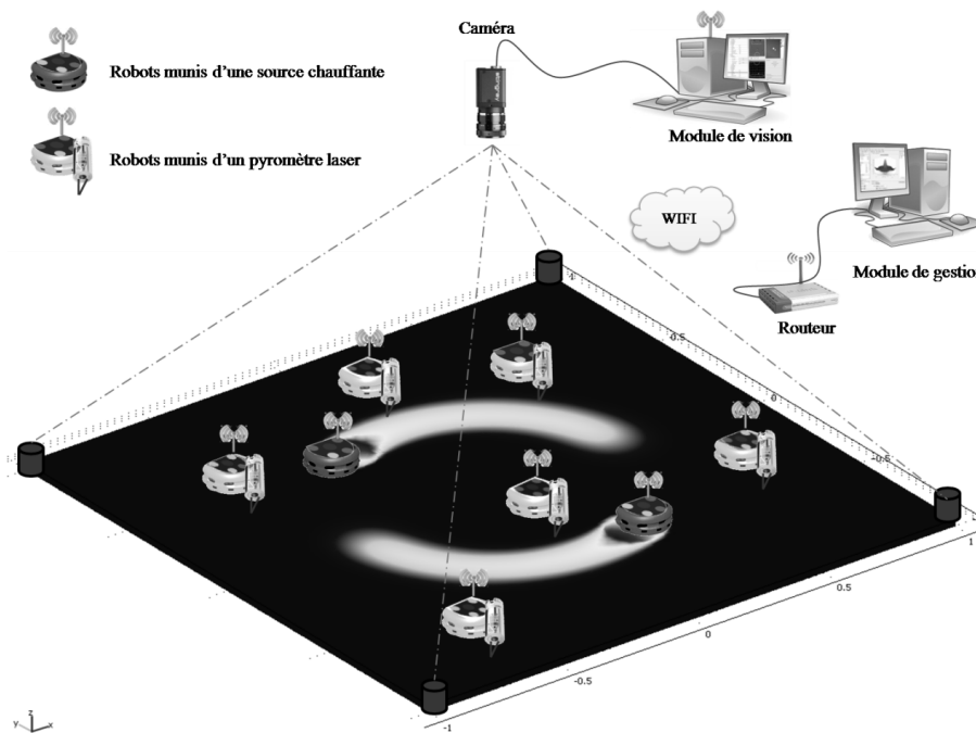
Figure 1 : Prototype du système de vision
