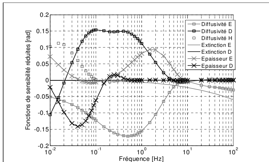
Figure 6. Fonctions de sensibilité réduites
